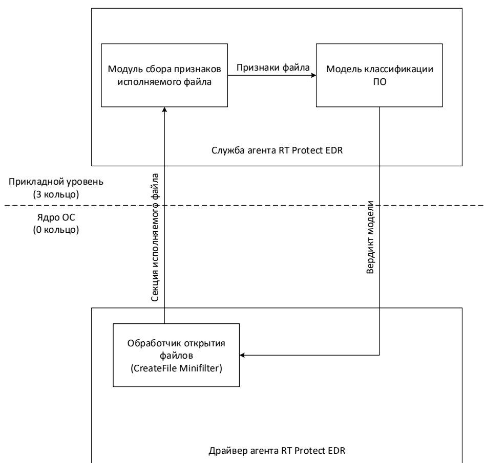
Рисунок 108 – Схема применения модели классификации ПО
