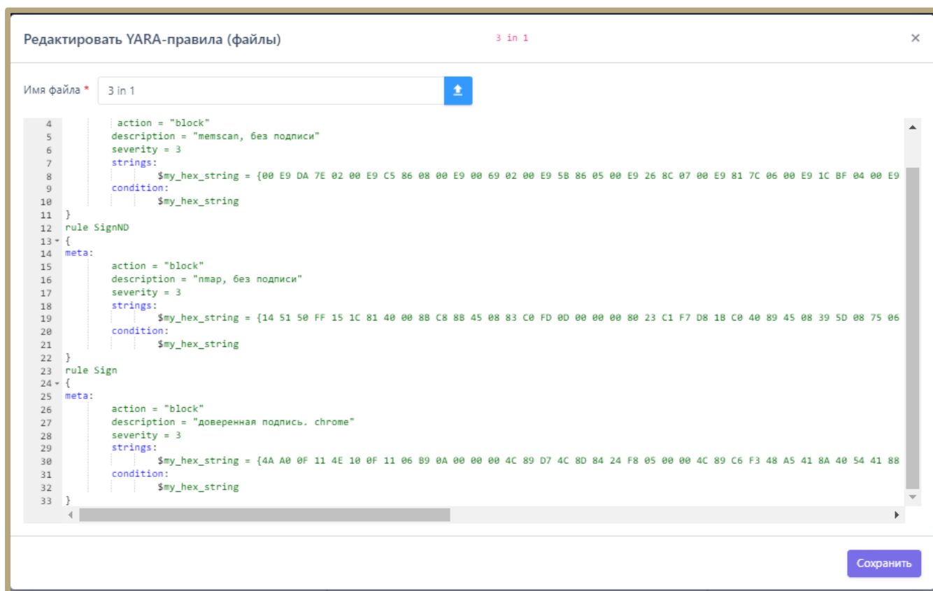
Рисунок 78 – Пример правила YARA
