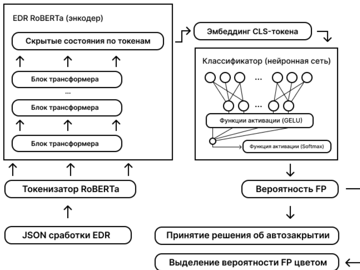
Рисунок 107 – Схема применения модели классификации инцидентов
