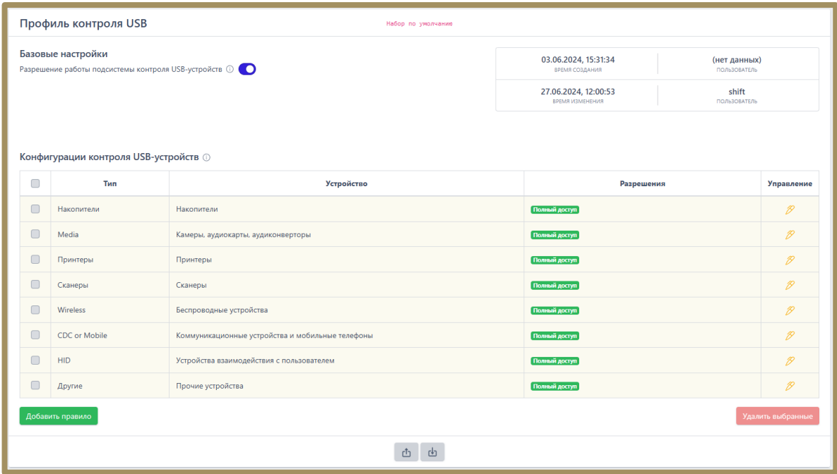
Рисунок 85 – Профиль контроля USB – Набор по умолчанию
